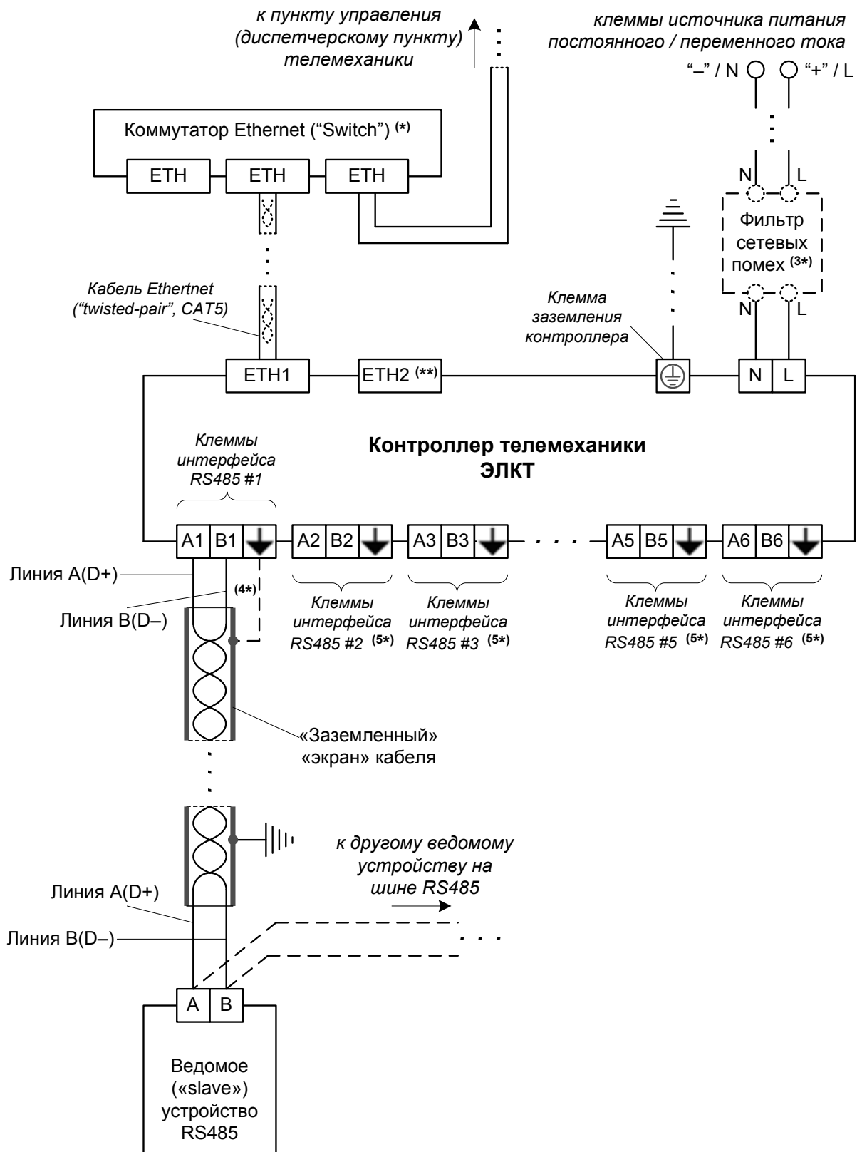
Рисунок Г.1 – Схема подключения контроллера (см. ниже примечания)
